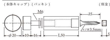
φ20×L50
