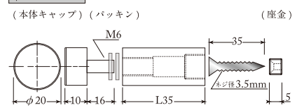
φ20×L35
