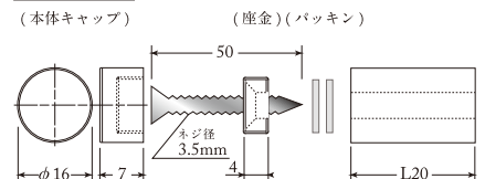
φ16×L20
