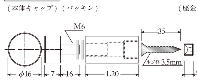
φ16×L20
