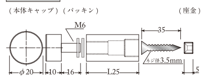
φ20×L25
